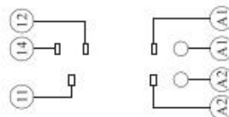
端子配置內部連接 Wiring Diagram
